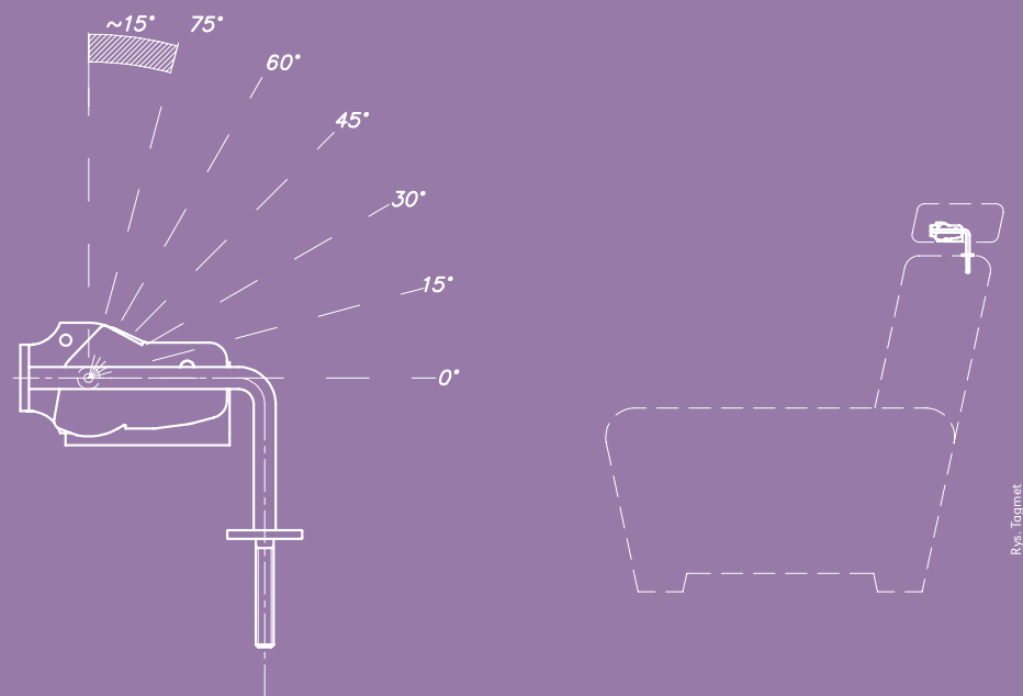
Zagłówek o wzmocnionej konstrukcji – ZG-016.01.
