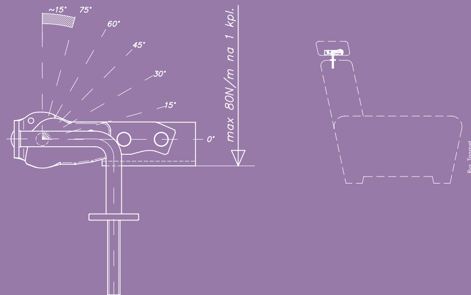
Mechanizm zagłówek z możliwością regulacji kąta oparcia – ZG-017.01
